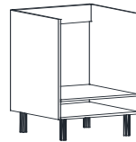
Mueble placa de cocción (sin trasera) Stove cupboard (without back)
